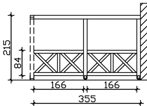
Bemassung
