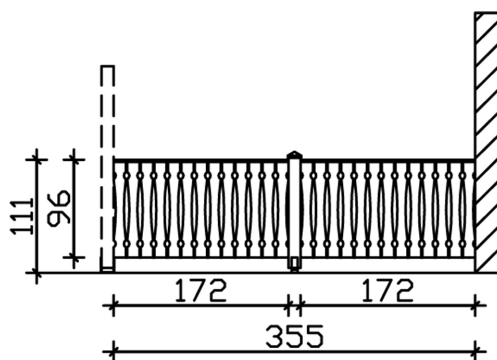
Bemassung
