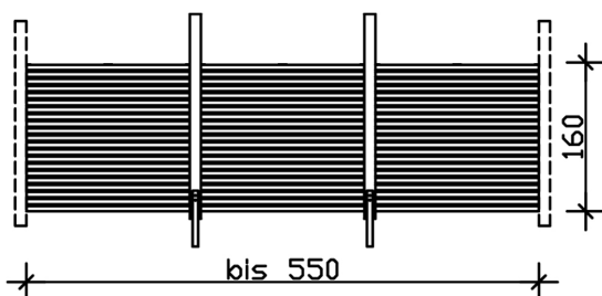
Bemassung
