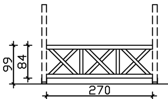
Bemassung
