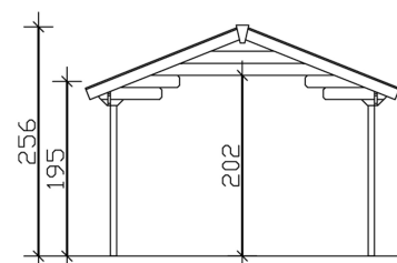
Schnitt
