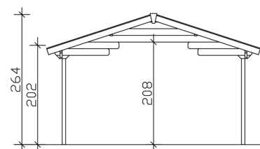
Schnitt
