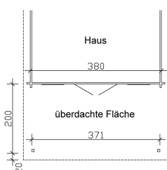
Grundriss
