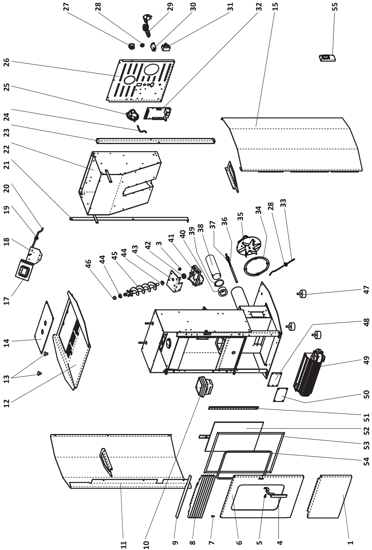
Abb. 14 Explosionszeichnung
