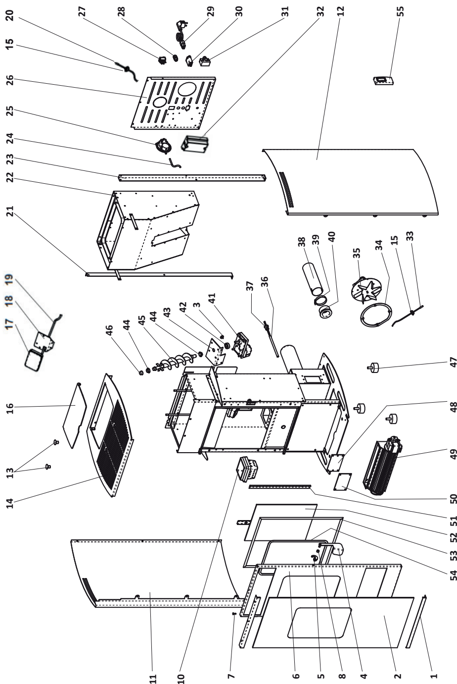
Abb. 14 Explosionszeichnung
