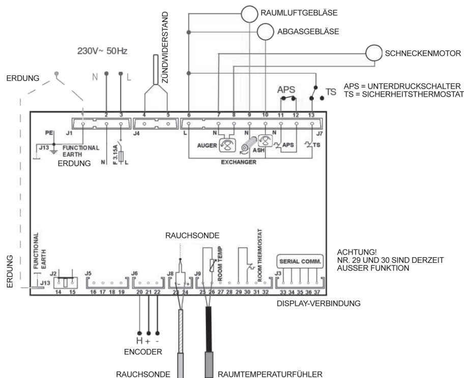
Abb. 15: Schaltplan der Platine
