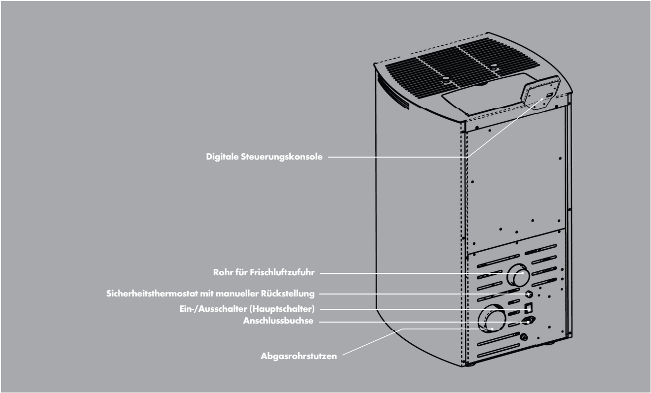
Abb. 1a: Geräteübersicht (Abbildung modellabhängig)
