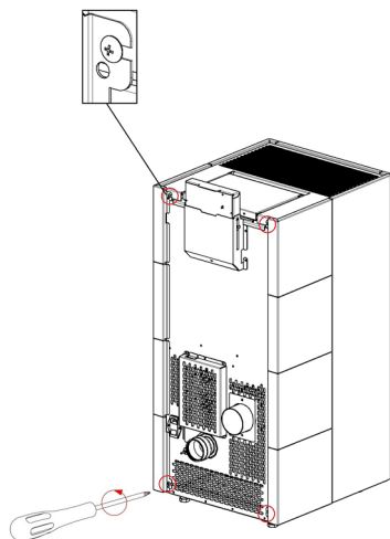
Fig. 57 - Schrauben lösen
