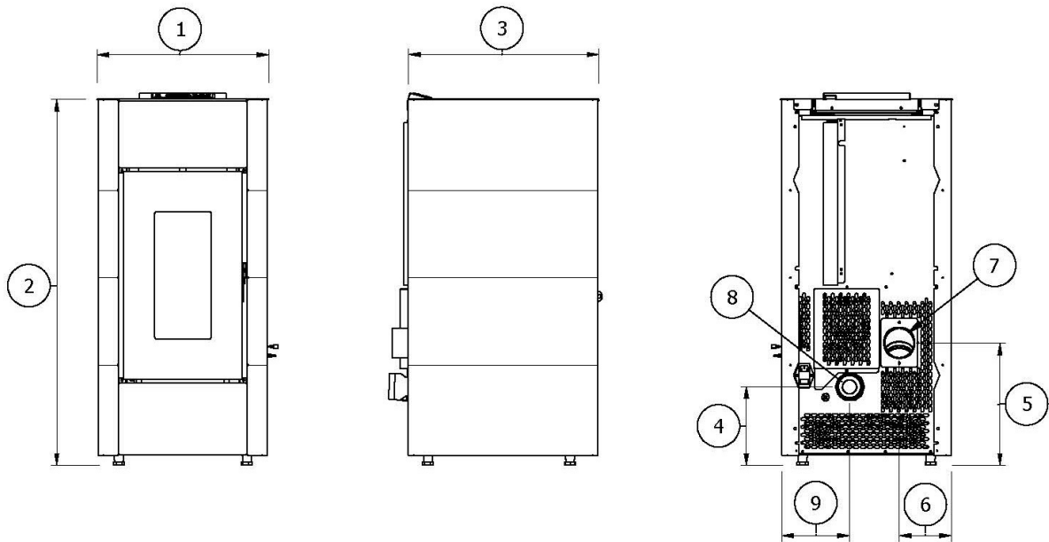
Fig. 23 - Allgemeine Abmessungen: Cristal³
