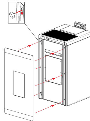
Fig. 37 - Das Glas positionieren
