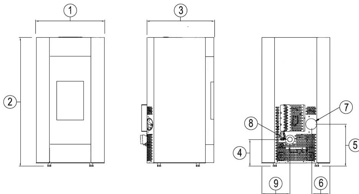
Fig. 20 - Allgemeine Abmessungen: Shell³
