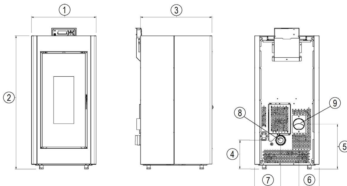
Fig. 22 - Allgemeine Abmessungen: Verve Airtight
