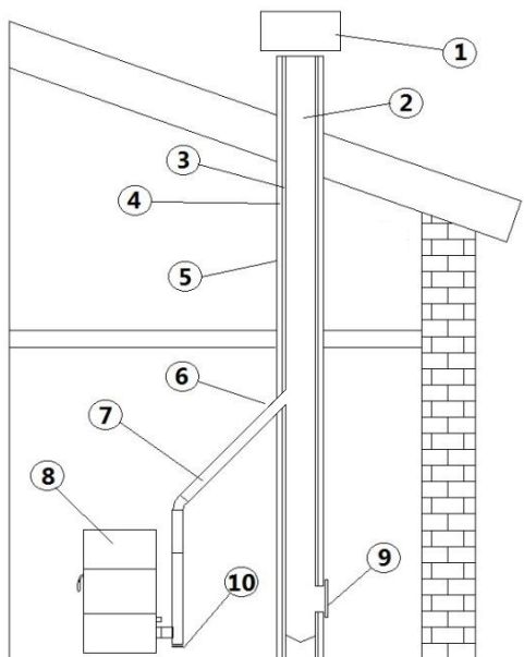
Fig. 6 - Bauteile Kamin
