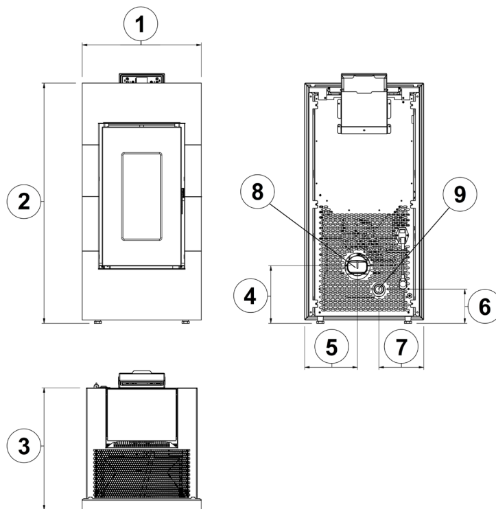
Fig. 16 - Allgemeine Abmessungen: KAMI evo
