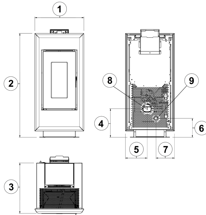
Fig. 17 - Allgemeine Abmessungen: ELAN evo
