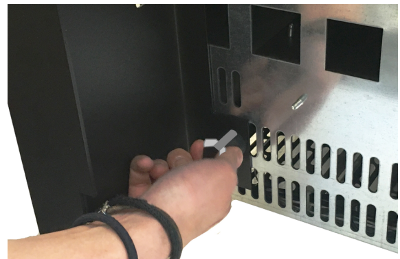
Fig. 30 - Den Sockel befestigen
