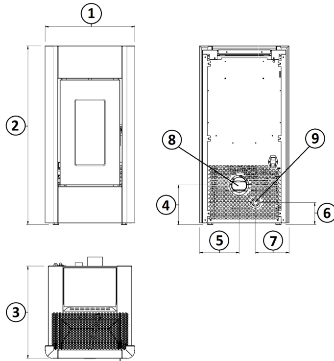
Fig. 14 - Allgemeine Abmessungen: SWEET
