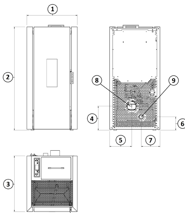
Fig. 13 - Allgemeine Abmessungen: FREE/LUNA
