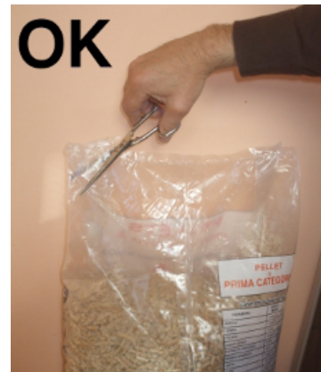
Fig. 35 - Korrekte Öffnung des Pelletsacks
