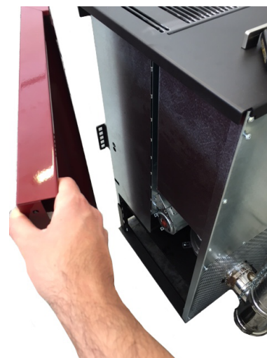
Fig. 21 - Entfernen der Seiten
