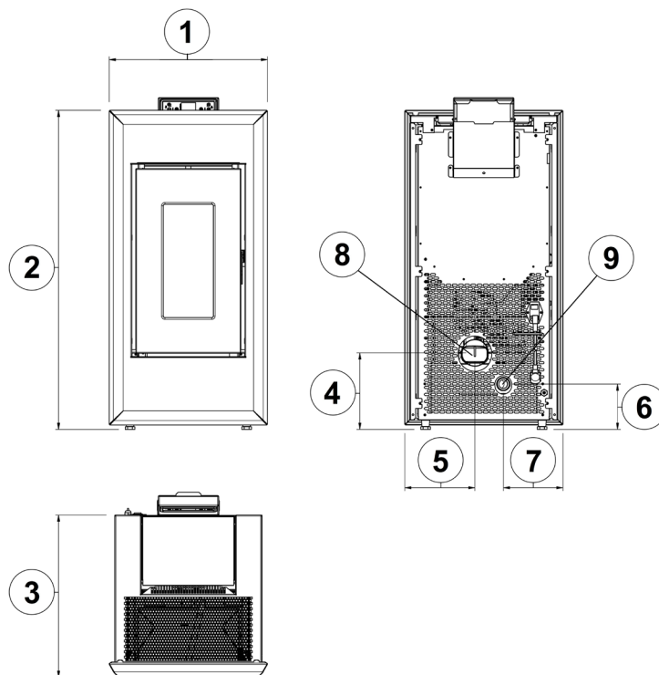
Fig. 15 - Allgemeine Abmessungen: MIKA evo
