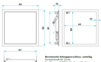
Revisionstür Schnappverschluss - einteilig Durchschnitt B3 32 mm Bauflugsmaß (BOM) A1 +5 mm / B1 +5 mm Revisionstür Schnappverschluss - 4-teilig Durchschnitt A3 13 mm Bauflugsmaß (BOM) A1 +5 mm / B1 +5 mm
