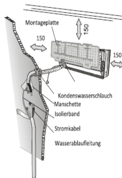
einzuhaltender Mindestabstand (mm) in der Abbildung
