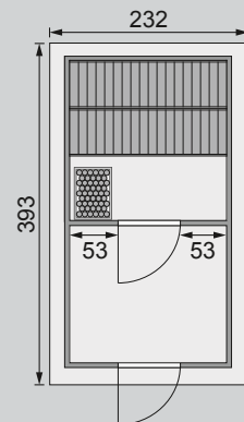
Dachstand / Innenaufteilung (in cm)
