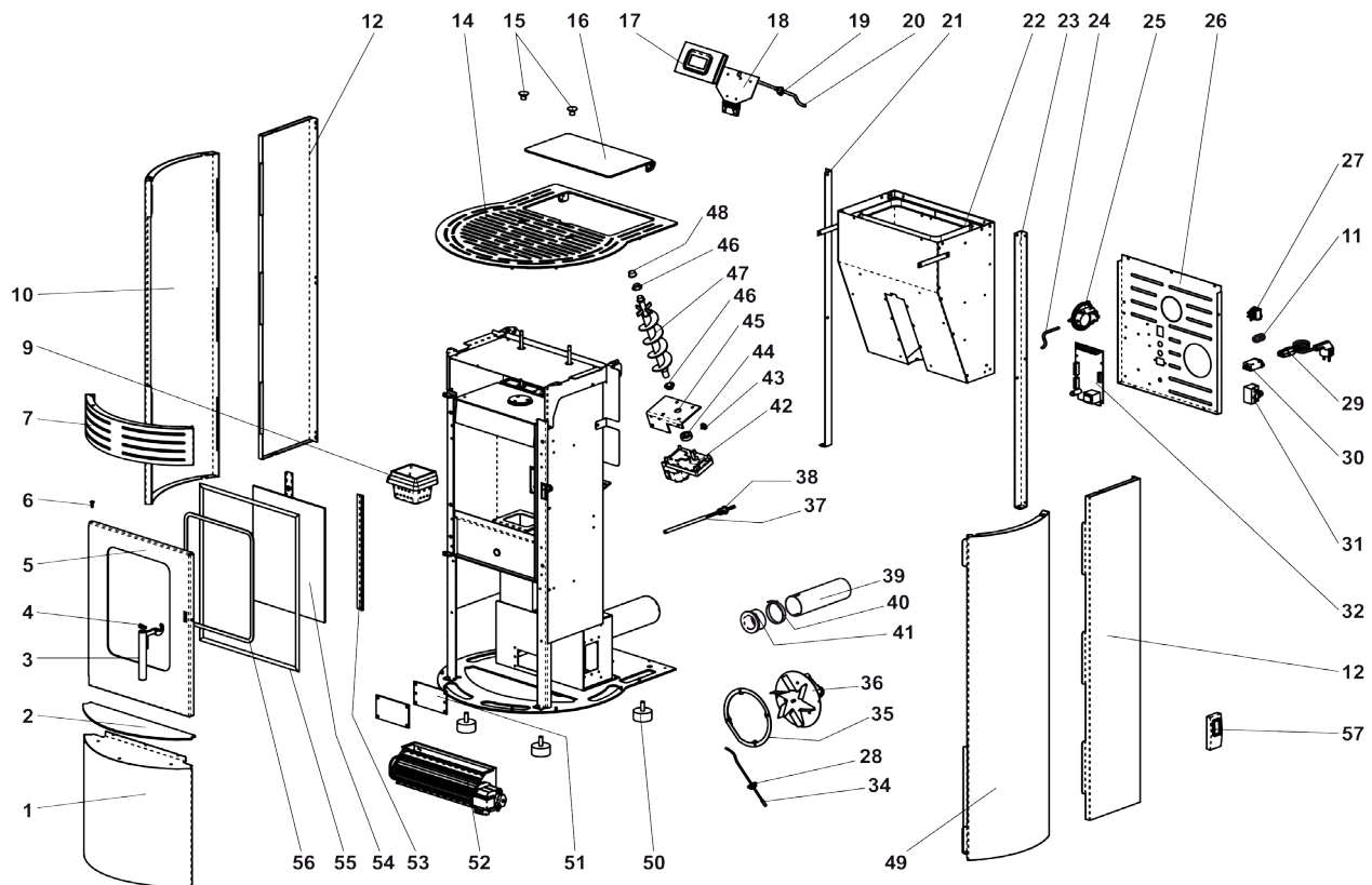
Abb. 15: Explosionszeichnung
