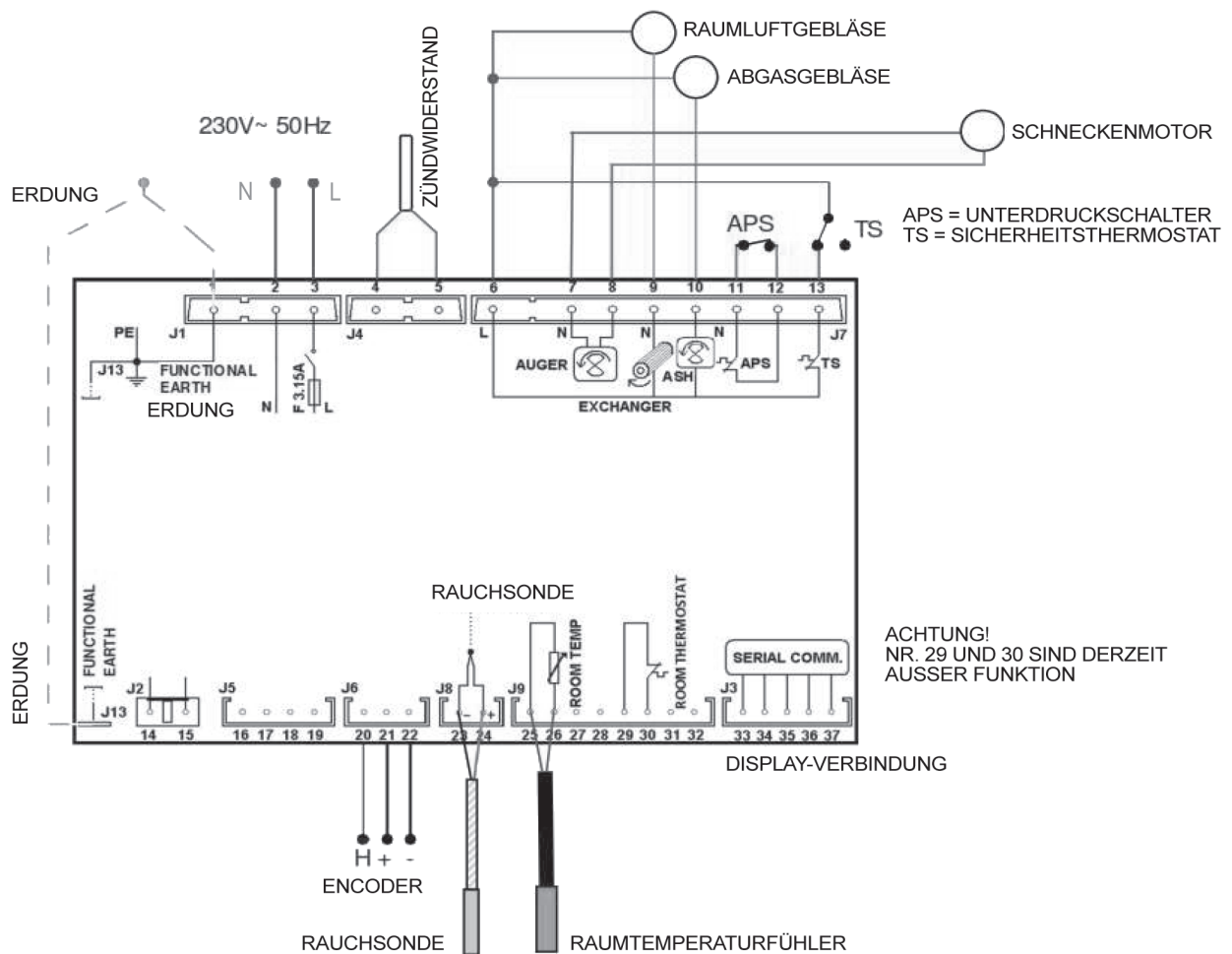
Abb. 16: Schaltplan der Platine
